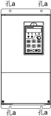
图 3-5 壁挂式安装示意图
