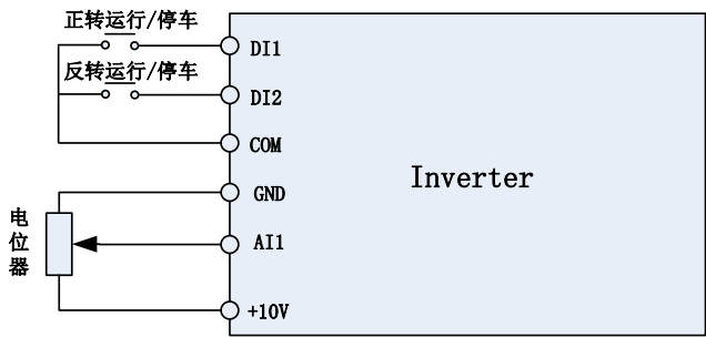
图 4 控制端子接线
