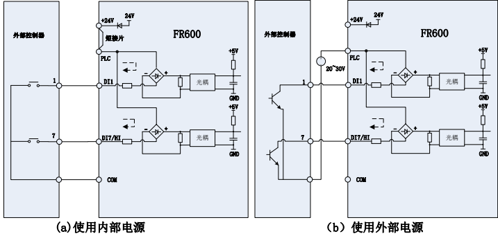
图 3-12 干接点方式
