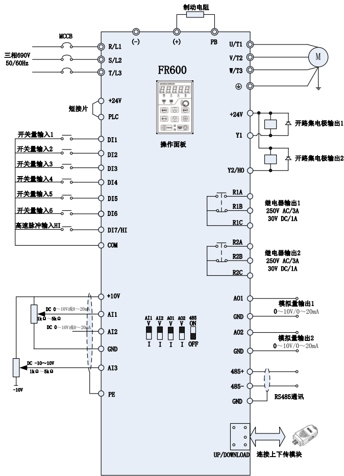
图 3-7 FR600 变频器接线示意图
