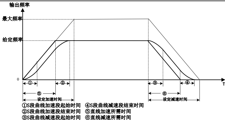
图 6-6 S 曲线加速减速示意图
