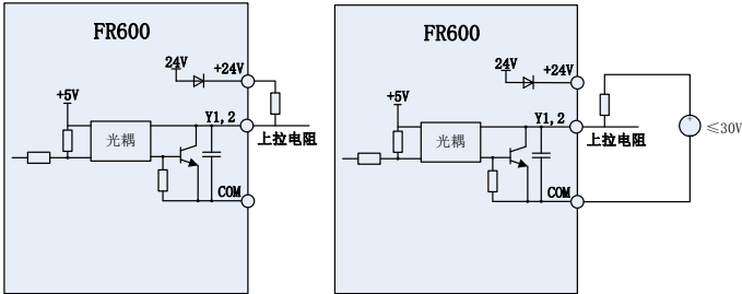
(a) 使用内部电源 (b) 使用外部电源 图 3-15 端子接上拉电阻输出时的接线方式
