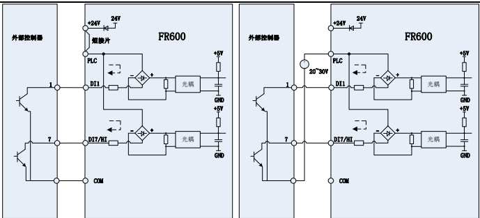
(a) 使用内部电源 (b) 使用外部电源 图 3-13 开路集电极 NPN 接线方式
