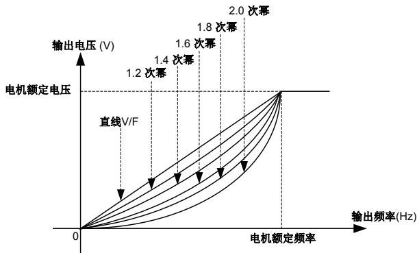
图 6-24 VF 曲线示意图
