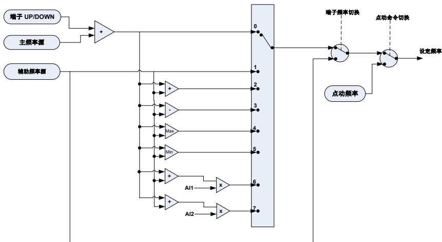
图 6-1 频率给定示意图
