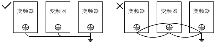
图 3-17 变频器接地处理
