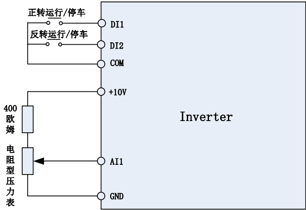
图 5 控制接线
