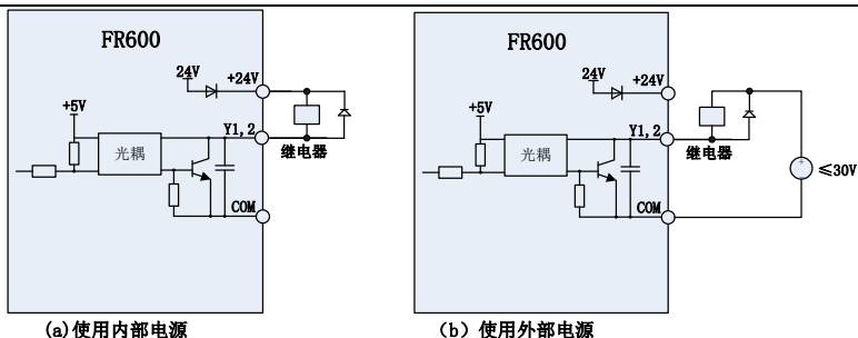
图 3-16 端子驱动继电器时的接线方式
