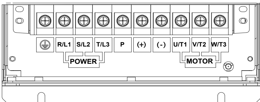
图 3-9 110~630kW 主回路端子示意图
