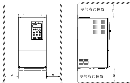
图 3-2 单台变频器安装方向及空间
