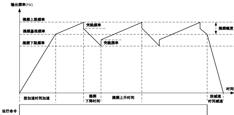
图 6-34 摆频功能示意图
