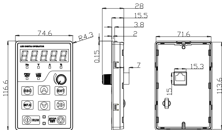
图 2-7 5.5~630KW 操作键盘尺寸图
