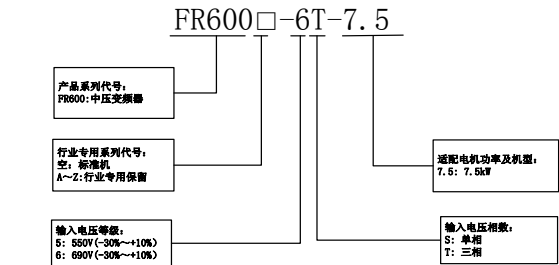
图 1 产品型号命名规则
