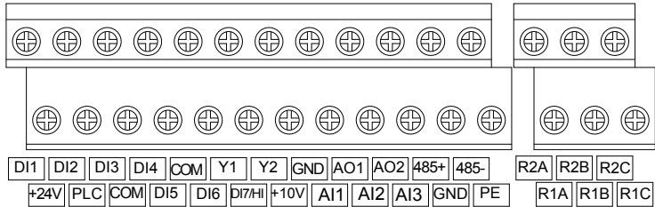
图 3 FR600 系列控制端子示意图
