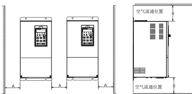
图 3-3 多台变频器并排安装方向及空间
