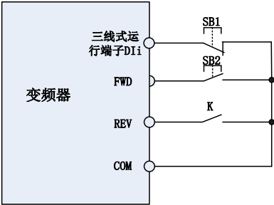
图 6-11 三线模式 2 控制示意图
