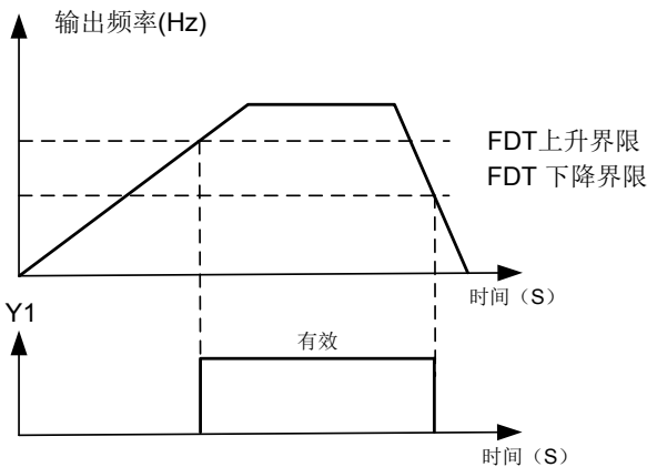
图 6-15 FDT 功能示意图
