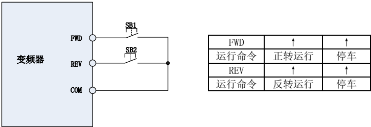
图 6-12 脉冲运行停车控制示意图
