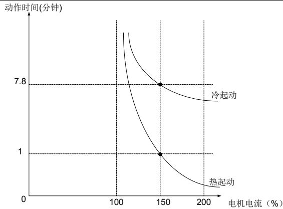
6-29 电机过载保护动作时间示意图
