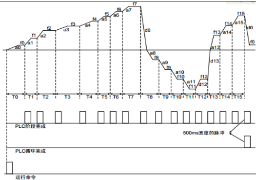
图 6-32 PLC 连续循环示意图
