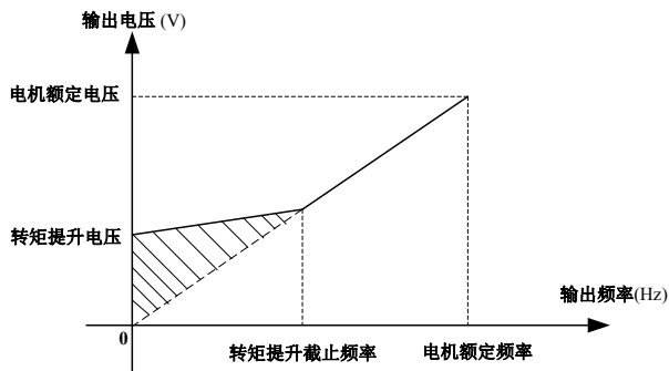
图 6-25 转矩提升示意图
