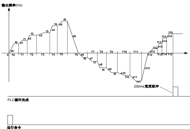
图 6-31 PLC 单循环后保持最终值示意图
