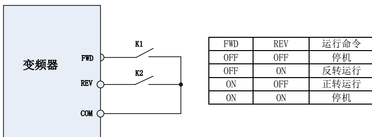
图 6-8 两线模式 1 控制示意图
