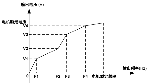
图 6-26 多点 VF 曲线示意图
