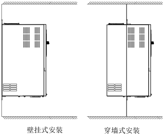
图 3-1 安装方式
