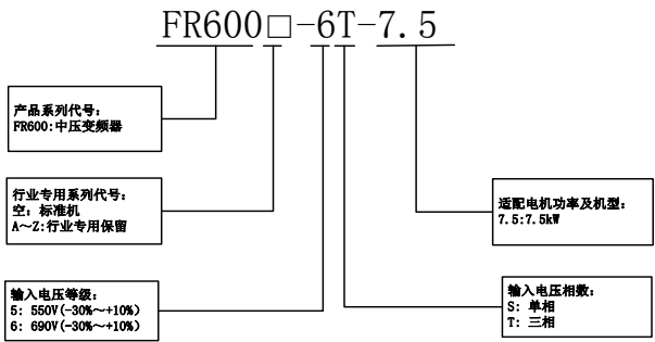
图 2-2 产品型号命名规则
