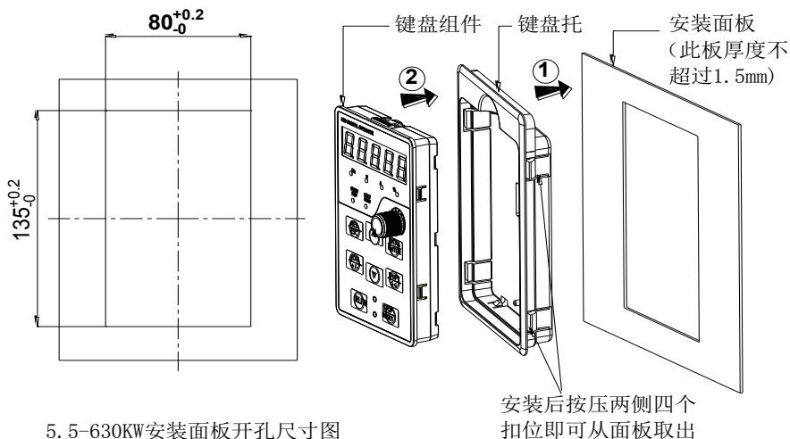
5.5~630KW 安装面板开孔尺寸图
