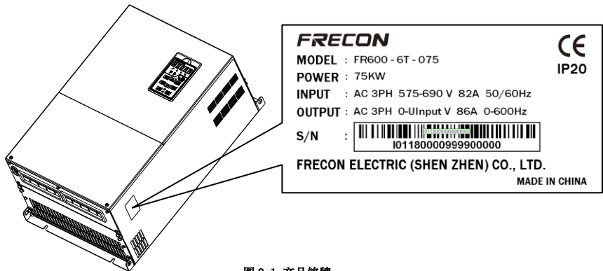
图 2-1 产品铭牌
