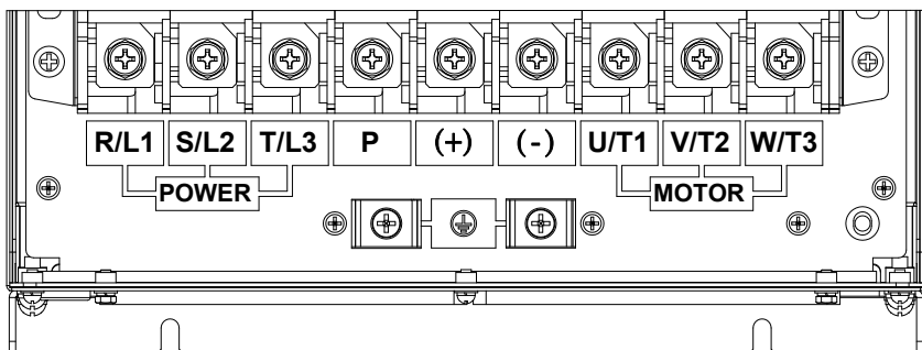
图 3-8 15~90kW 主回路端子示意图
