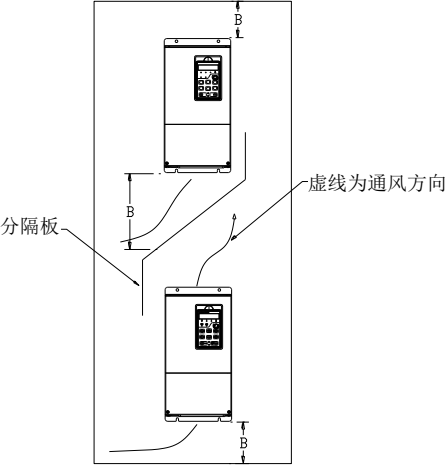
图 3-4 多台变频器上下安装方向及空间 表 3-1 变频器安装空间要求
