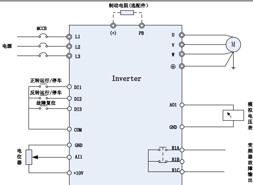
图 6 整体接线
