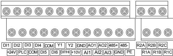
图 3-10 控制端子示意图 表 3-3 FR600 变频器控制回路端子功能
