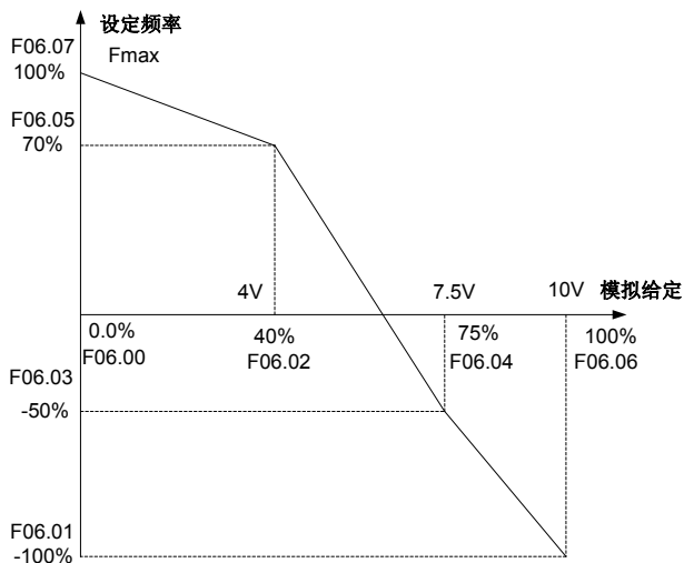
图 6-17 (2) 代码参数设定示意图
