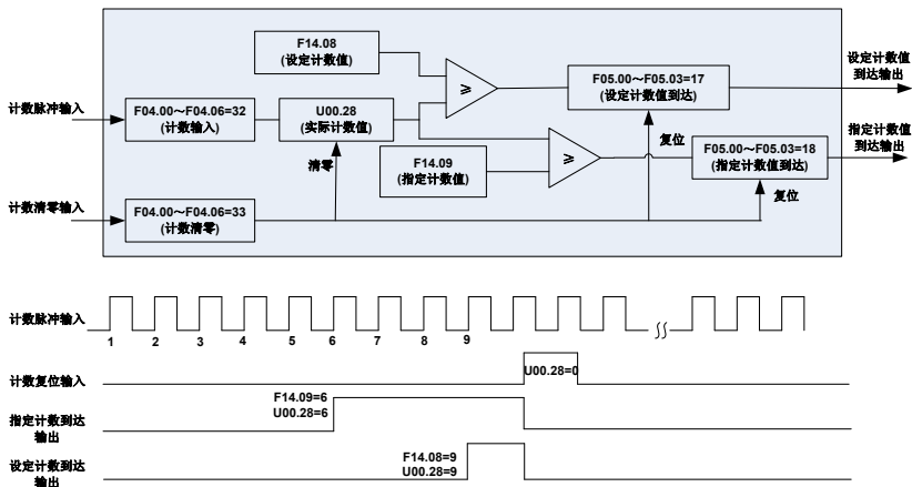
图 6-36 计数功能示意图
