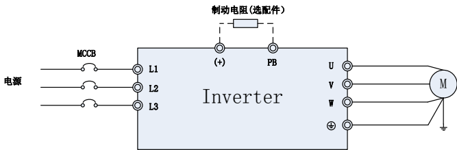
图 2 主回路接线
