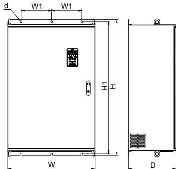
图 2-5 220~630kW 壁挂安装示意图(2)
