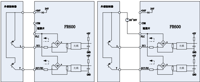
(a) 使用内部电源 (b) 使用外部电源 图 3-14 开路集电极 PNP 接线方式
