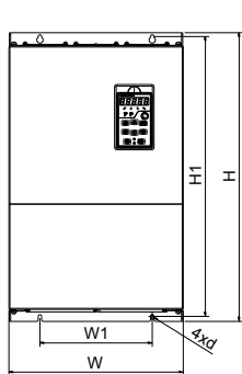
图 2-4 15~200kW 壁挂安装示意图(1)
