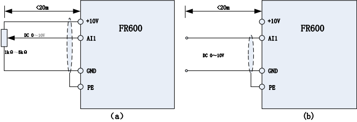
图 3-11 模拟量输入端子接线示意图
