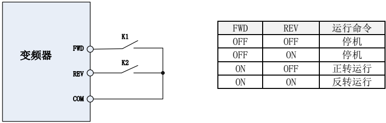
图 6-9 两线模式 2 控制示意图
