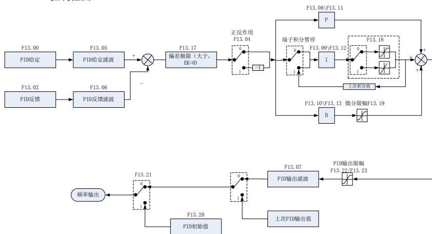
图 6-33 PID 控制框图
