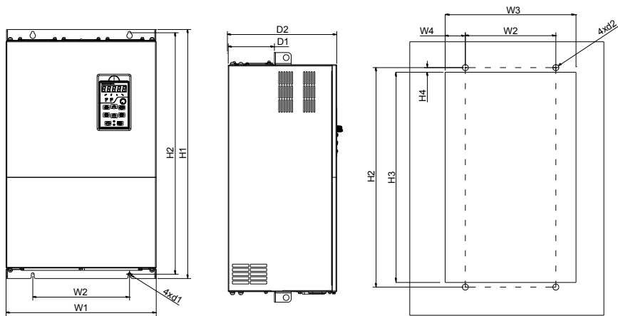
图 2-6 5.5~200kW 穿墙安装示意图 表 2-4 穿墙安装尺寸表
