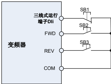
图 6-10 三线模式 1 控制示意图
