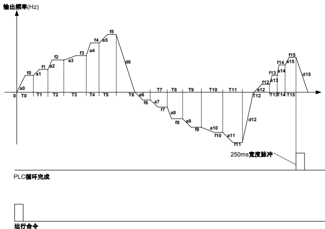
图 6-30 PLC 单循环后停机示意图
