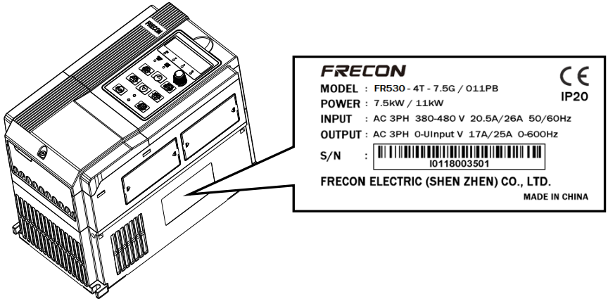
图 1-1 产品铭牌
