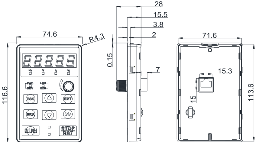
图 c-2 7.5~450kW 操作键盘尺寸图
