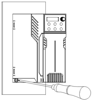
图 3-6(e) 壁挂安装示意图
