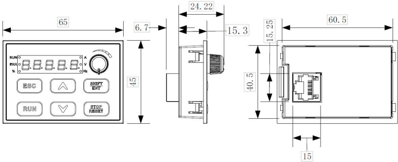
图 2-3 操作键盘尺寸图
