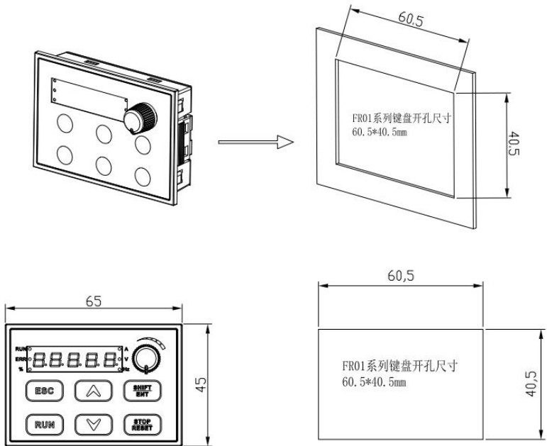
图 2-3 操作键盘尺寸图
