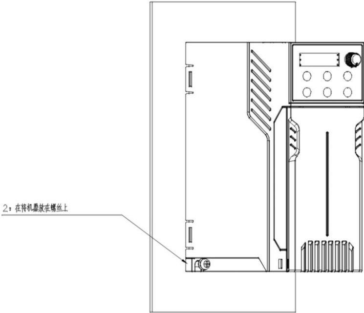
图 3-6(b) 壁挂安装示意图
