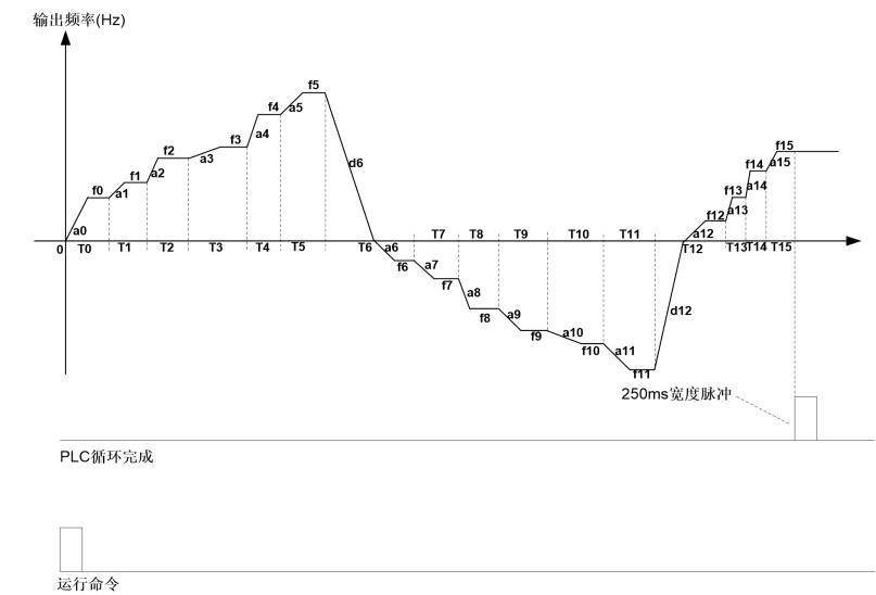
图 6-31 PLC 单循环后保持最终值示意图
