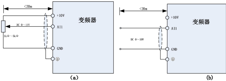
图 3-19 模拟量输入端子接线示意图
