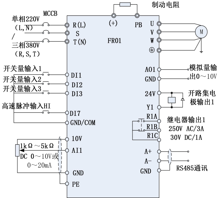
图 3-10 FR01 变频器接线示意图
