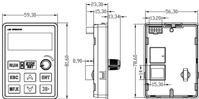
图 2-4 LCD 选配键盘（带参数拷贝）（申购编码：02.35.0077）
