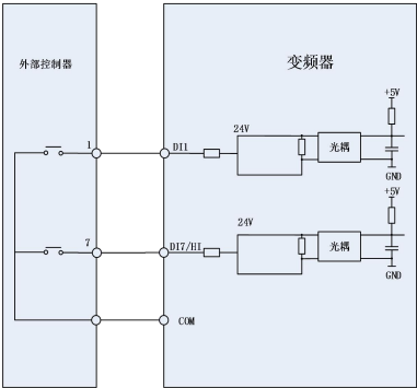
(a) 使用内部电源 图 3-20 干接点方式
