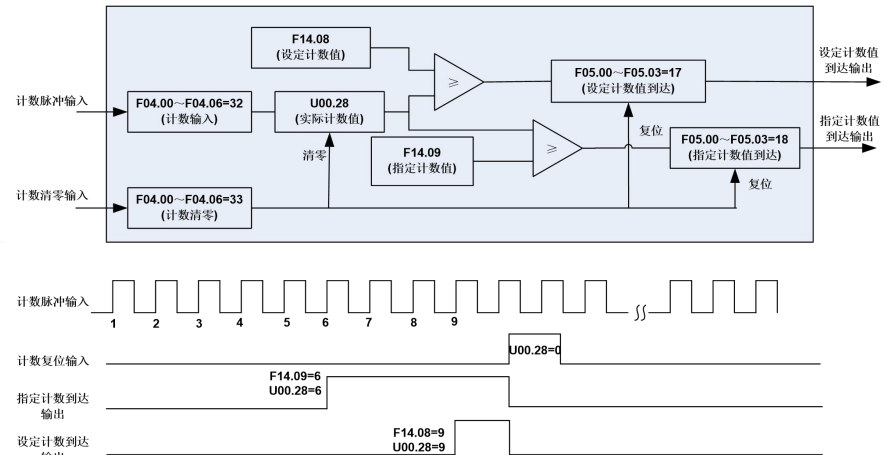
图 6-36 计数功能示意图
