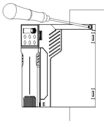
图 3-6(d) 壁挂安装示意图
