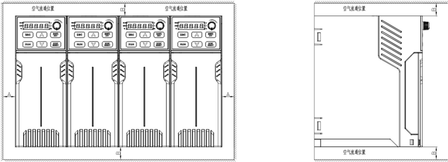
图 3-2 多台变频器并排安装方向及空间
