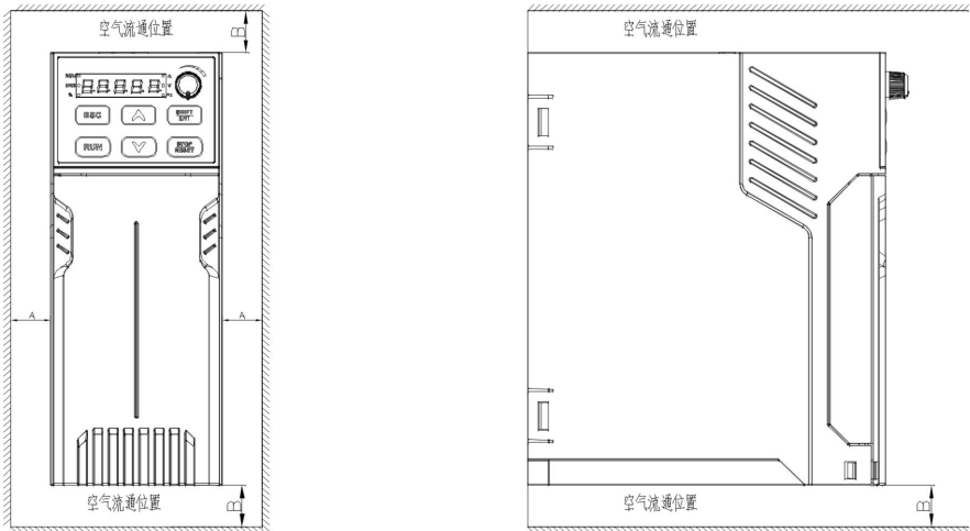
图 3-1 单台变频器安装方向及空间
