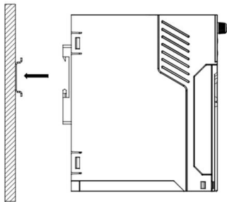
图 3-7(b) 导轨式安装示意图
