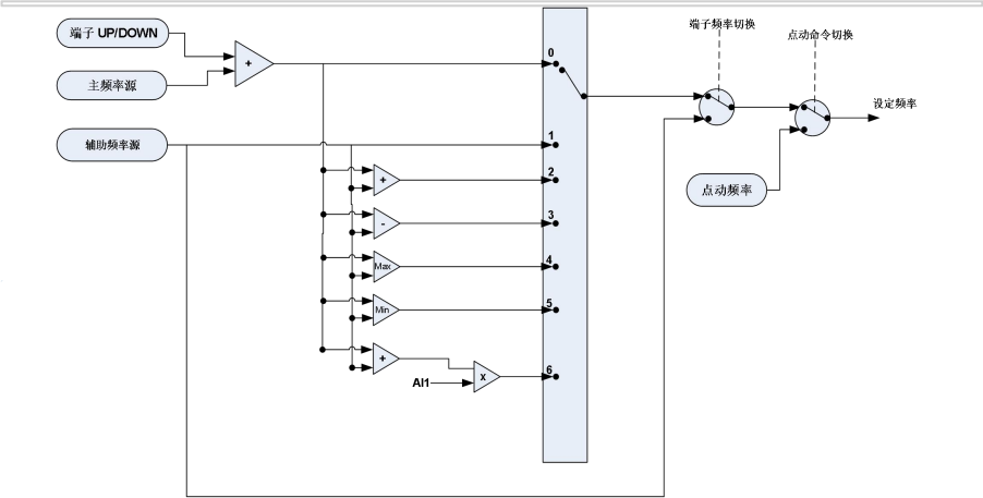
图 6-1 频率给定示意图
