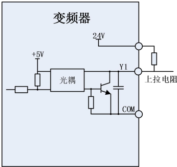
(a) 使用内部电源 图 3-19 端子接上拉电阻输出时的接线方式
