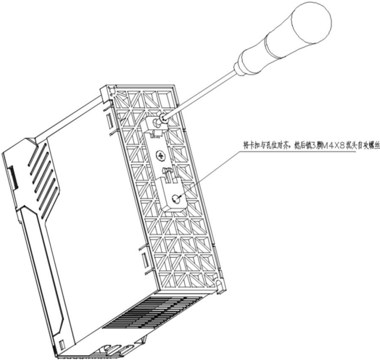
图 3-7(a) 导轨式安装示意图
