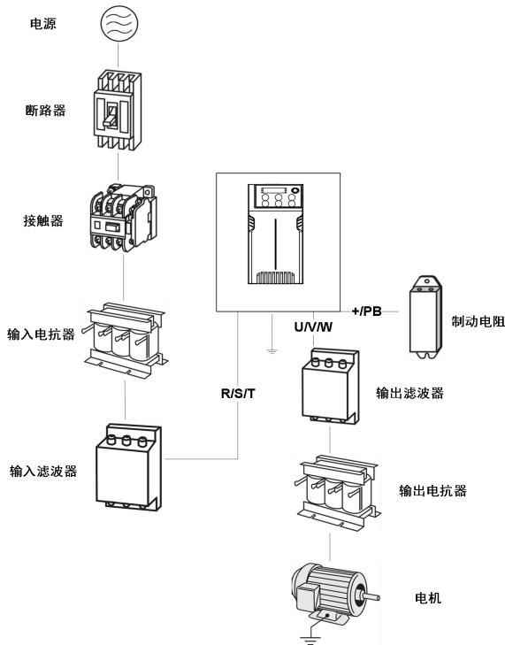
图 3-10 产品外围器件及配线
