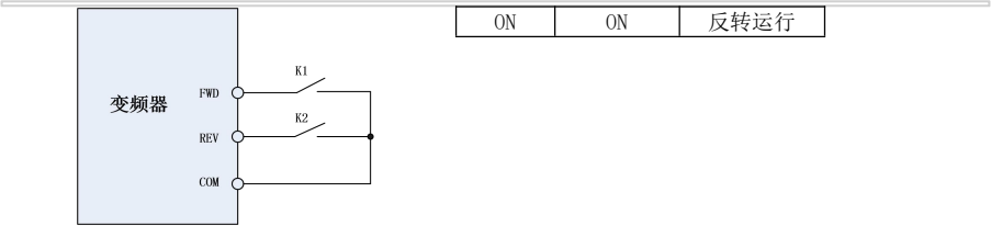
图 6-9 两线模式 2 控制示意图
