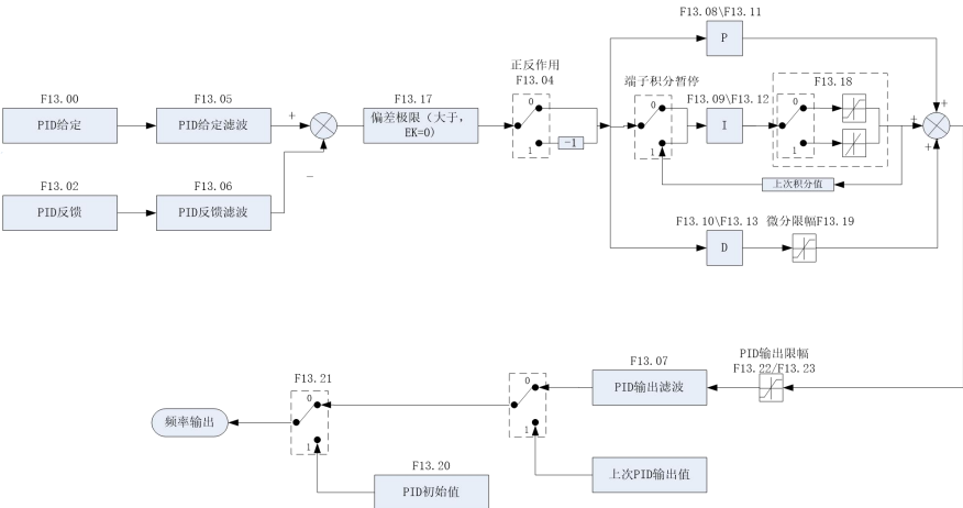
图 6-33 PID 控制框图
