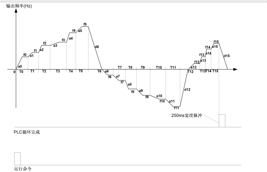
图 6-30 PLC 单循环后停机示意图
