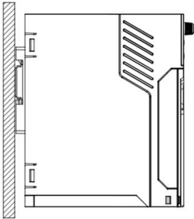
图 3-7(c) 导轨式安装示意图
