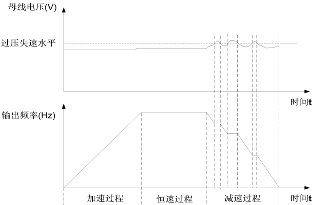
图 6-28 过压失速模式 1 示意图
