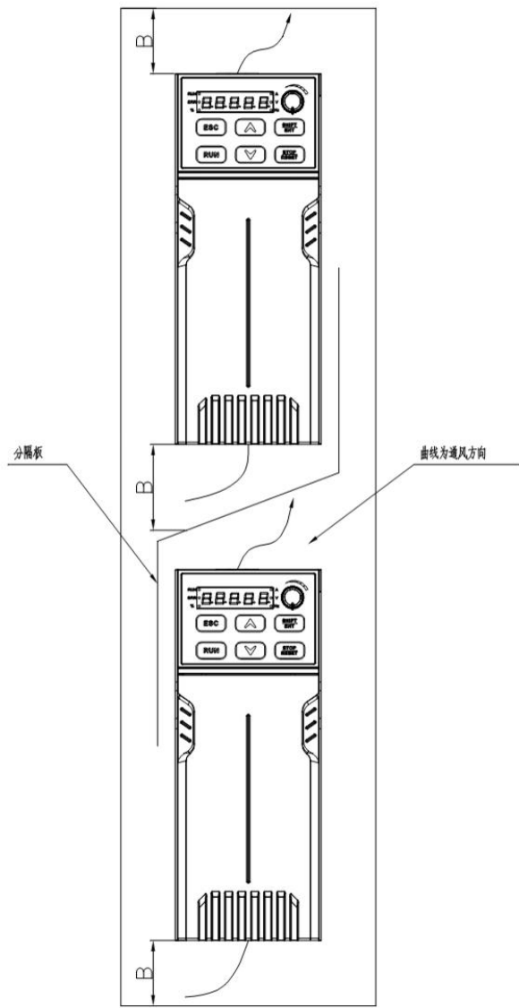
图 3-3 多台变频器上下安装方向及空间 表 3-1 变频器安装空间要求
