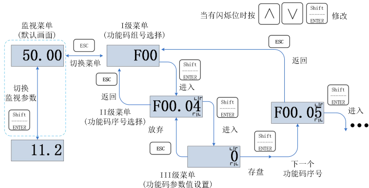
图 4-2 三级菜单操作流程
