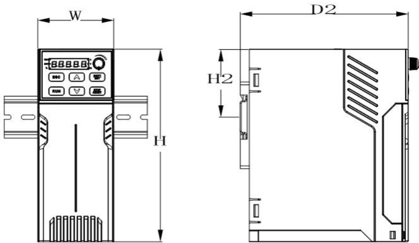
图 3-5 导轨安装尺寸
