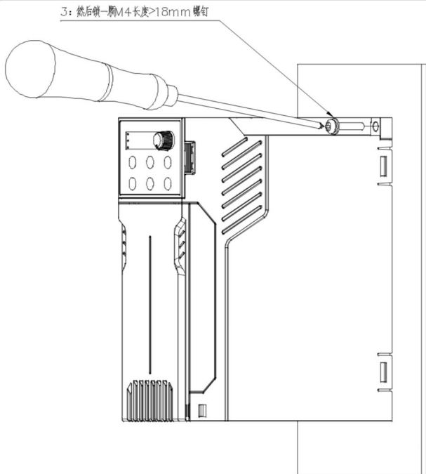
图 3-6(c) 壁挂安装示意图
