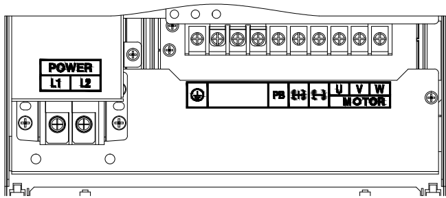
4.0-11KW 主回路端子
