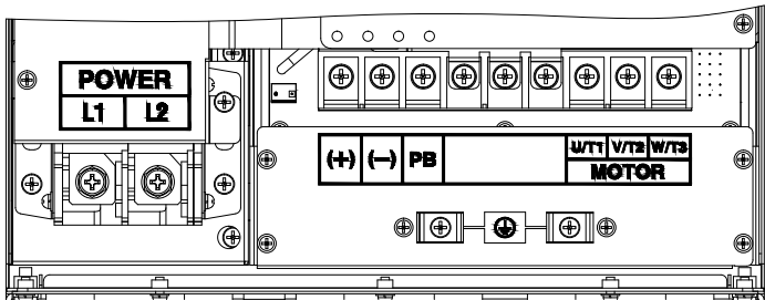
15-22KW 主回路端子
