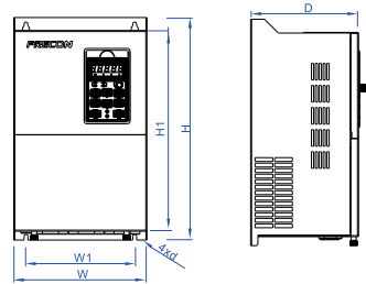
30-560Kw结构示意图
