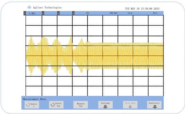
震荡抑制波形图
