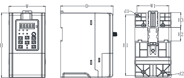
□ FR150A (0.2~22KW) 安装尺寸
