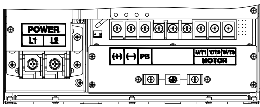
15-22kW 主回路端子
