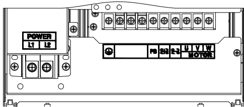
4.0-11kW 主回路端子
