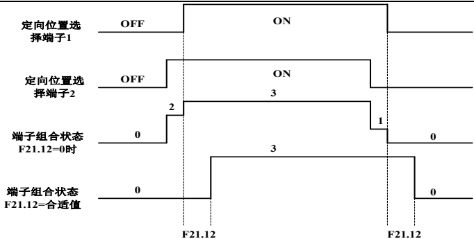
图 6-30 定向位置确认
