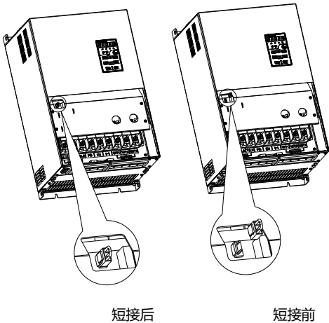
图 3-25 30kW 以上短接示意图
