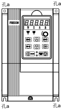
图 3-5 壁挂式安装示意图
