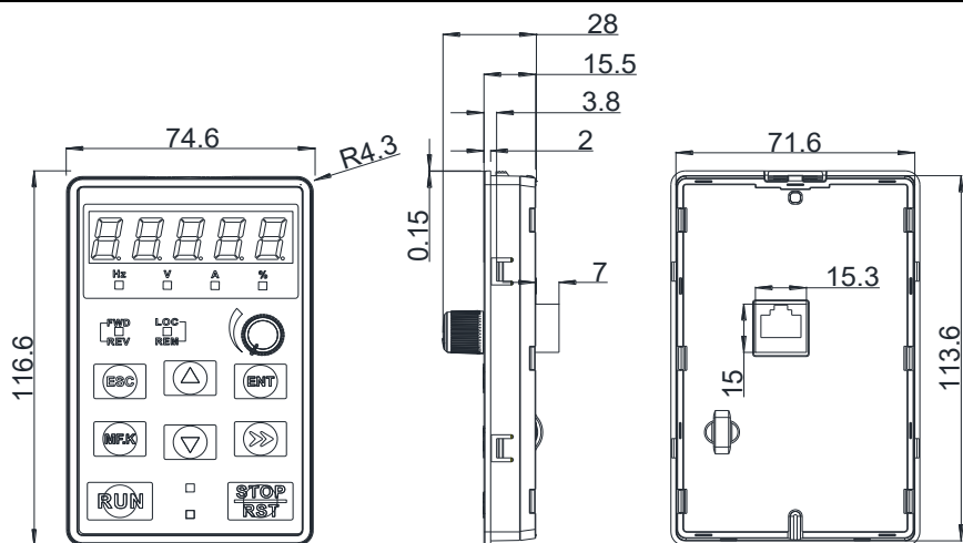
图 2-10 7.5~800kW 操作键盘尺寸图
