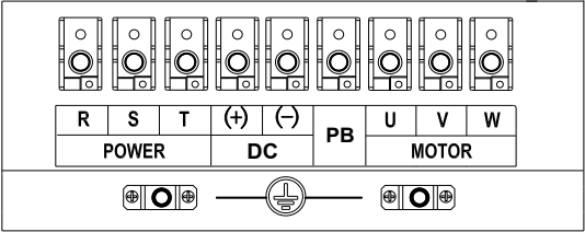
图 3-15 45~90kW 主回路端子示意图
