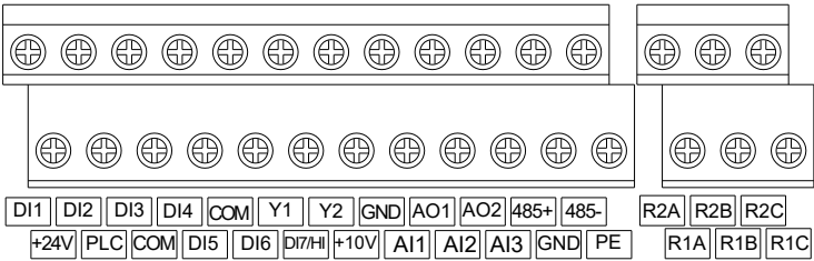
图 3-18b 控制端子示意图
