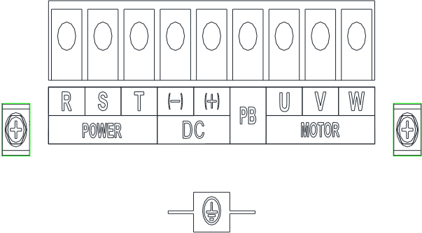
图 3-14 30~37kW 主回路端子示意图
