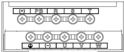
图 3-11 0.7 ~ 2.2kW 主回路端子示意图
