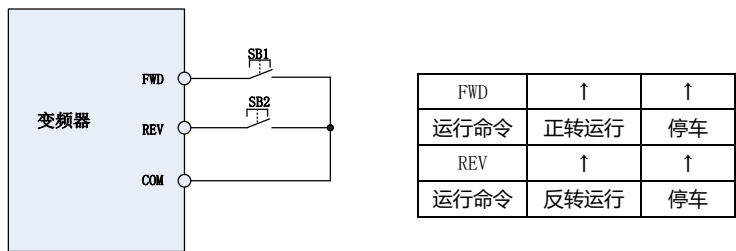
图 6-12 脉冲运行停车控制示意图
