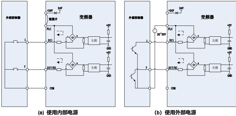
图 3-20 干接点方式
