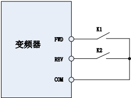
图 6-8 两线模式 1 控制示意图
