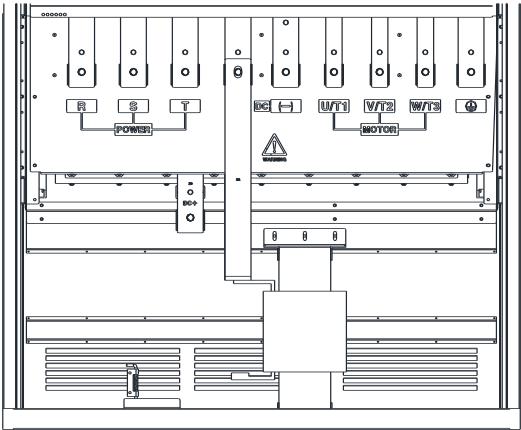
图 3-18 630 ~ 710kW 主回路端子示意图
