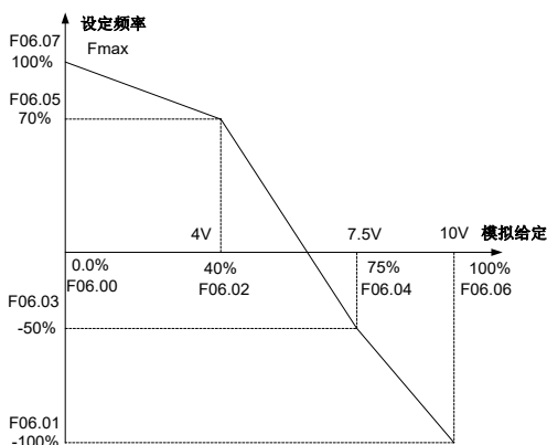
图 6-17 (2) 代码参数设定示意图
