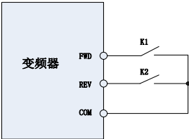
图 6-9 两线模式 2 控制示意图
