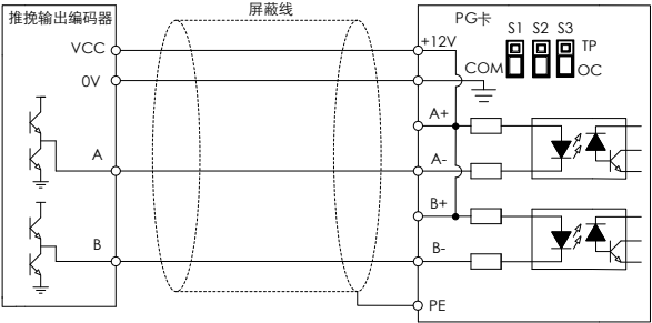
图 C-6 EXC-PG02 与推挽输出编码器连接示意图
