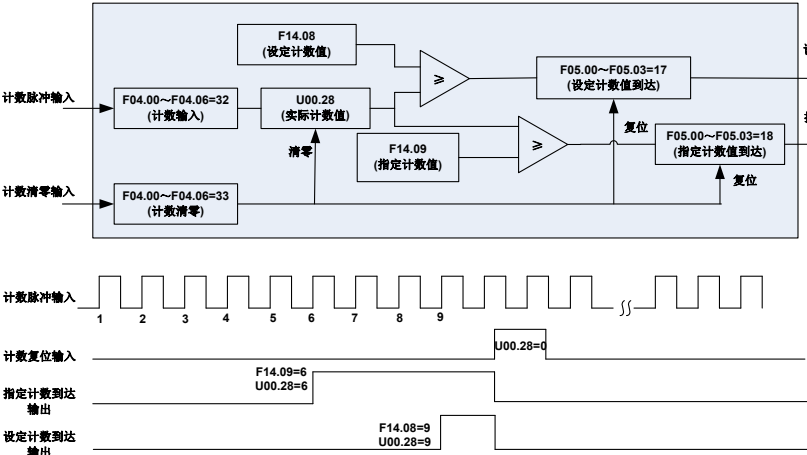
图 6-36 计数功能示意图
