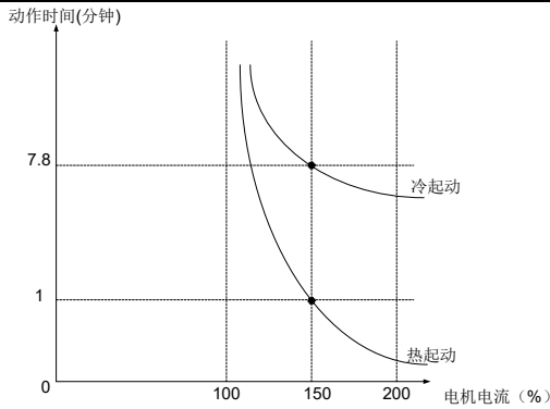
图 6-29 电机过载保护动作时间示意图
