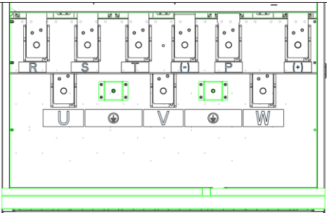
图 3-17 500 ~ 560kW 主回路端子示意图
