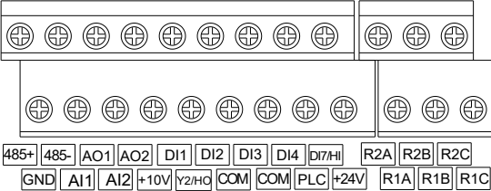
图 3-18a 控制端子示意图
