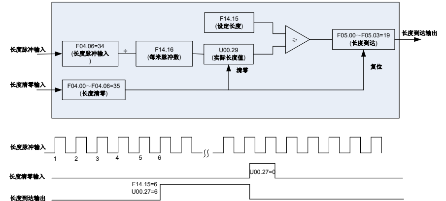
图 6-35 定长功能示意图
