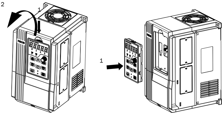
图 3-7(a) 操作面板拆卸示意图 3-7(b) 操作面板安装示意图
