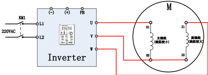
图 6-20 FR500&FR510 ( > 0.75\text{kW} ) 与单相电机正转接线图
