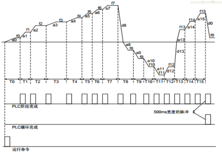
图 6-32 PLC 连续循环示意图
