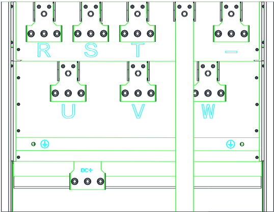
图 3-18 800 ~ 1120kW 主回路端子示意图
