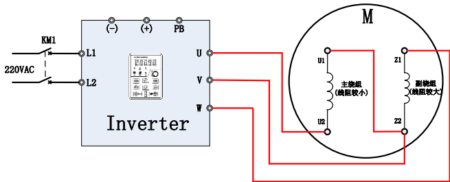
图 6-21 FR500&FR510 (> 0.75kW) 与单相电机反转接线图
