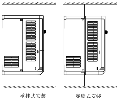
图 3-1 安装方式
