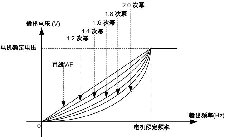
图 6-24 V/F 曲线示意图
