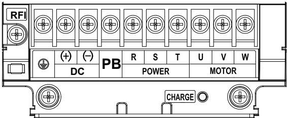
Fig.2-17b 2S 系列主回路端子(4.0~7.5kW)
