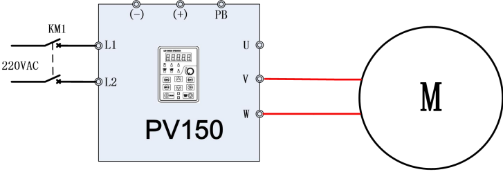
图 2-13 PV150 接线
