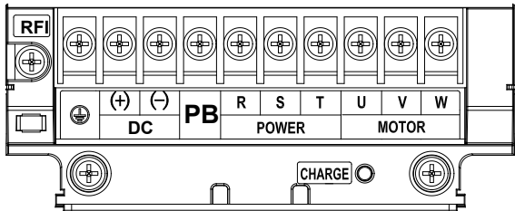
Fig.2-21 主回路端子 (7.5~22kW)
