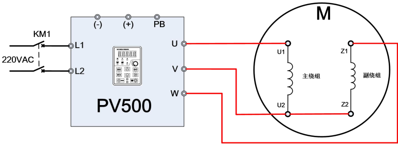
图 2-11 PV500 ( >0.75\text{kW} ) 与单相电机正转接线
