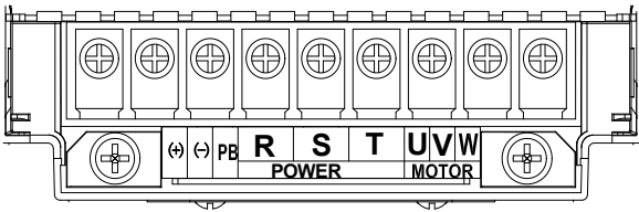
Fig.2-20 主回路端子 (4~5.5kW)
