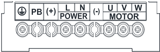
Fig.2-17a 2S系列主回路端子 (≤2.2kW)
