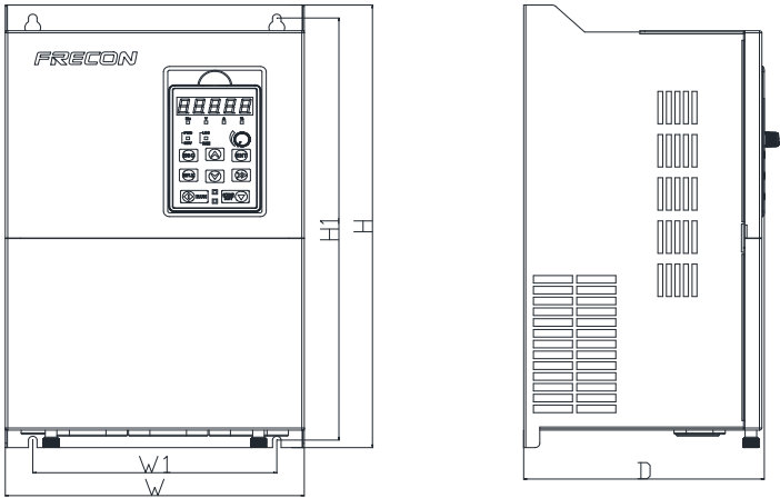
Figure 1-5 30~280kw 外形和安装尺寸
