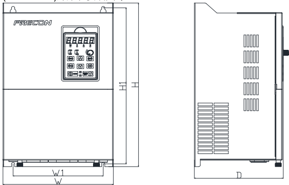
Fig 1-4 2T-18~75KW 外形和安装尺寸
