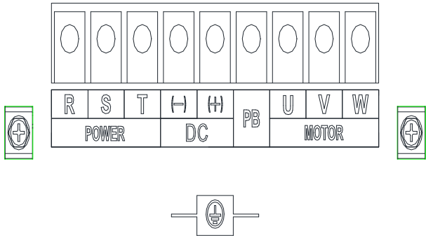
Fig.2-22 主回路端子 (30~37kW)
