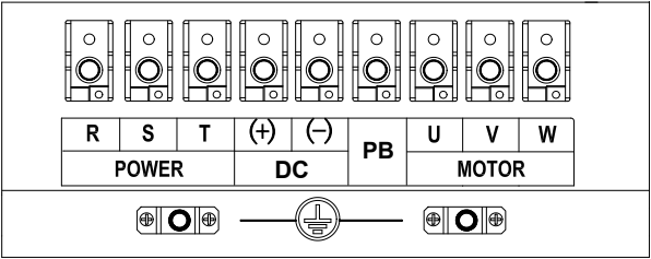
Fig.2-23 主回路端子（45~90kW）
