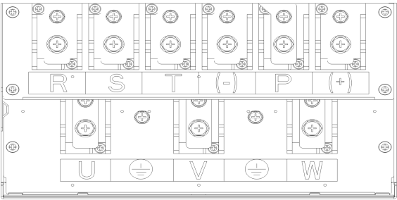
Fig.2-25 主回路端子（450~560kW）
