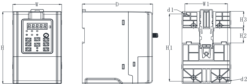
图 1-3 PV150 外形尺寸
