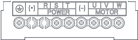
Fig.2-18a 主回路端子 (0.7~4.0kW)
