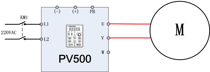
图 2-14 PV500 接线
