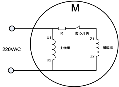
图 2-7 电阻启动模式:双电容电机内部接线
