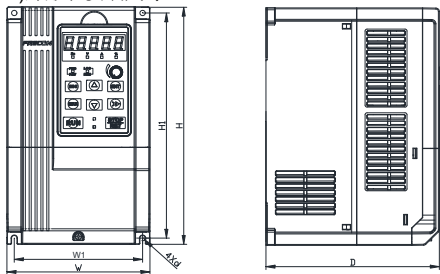
Fig 1-3 2T-4.0~11kW 外形和安装尺寸
