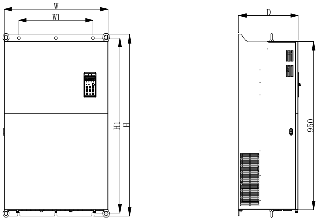
Figure 1-5 30~280kw 外形和安装尺寸
