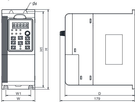
图 1-4 0.7~2.2kW 外形和安装尺寸
