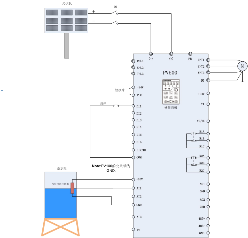
图 2-1 光伏电池供电时接线图
