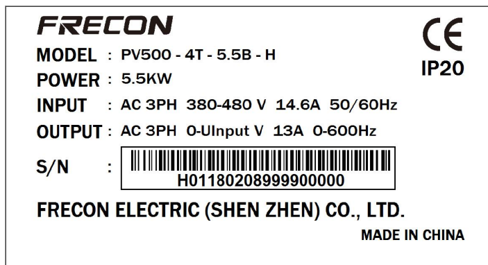
图 1-1 产品铭牌
