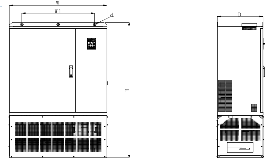
Figure 1-6 30~450kw 外形和安装尺寸
