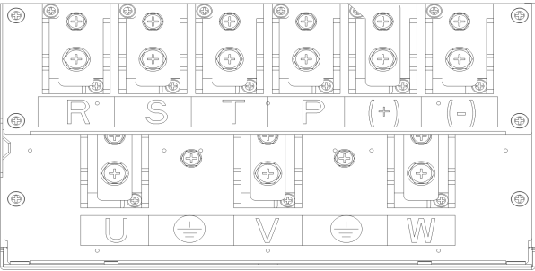
Fig.2-24 主回路端子（110~400kW）
