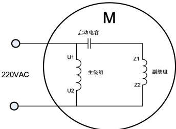
图 2-4 运行模式:单电容电机内部接线
