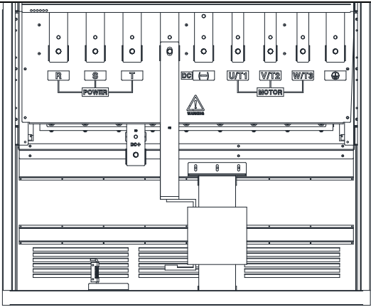
Fig.2-25 630~710KW 主回路端子
